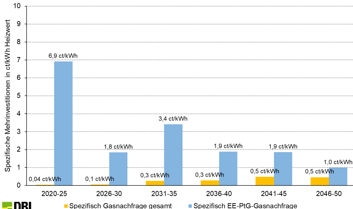
Spezifische erforderliche Mehrinvestitionen zur Treibhausgasneutralität der Gasnetze und Gasspeicher - Basis-Szenario
