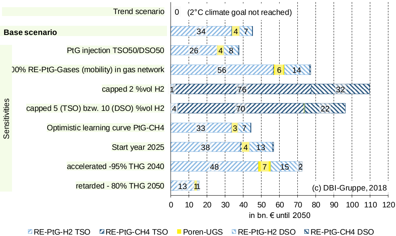
Transformationspfade Gasnetze und Gasspeicher - Mehrkosten in Mrd. €
