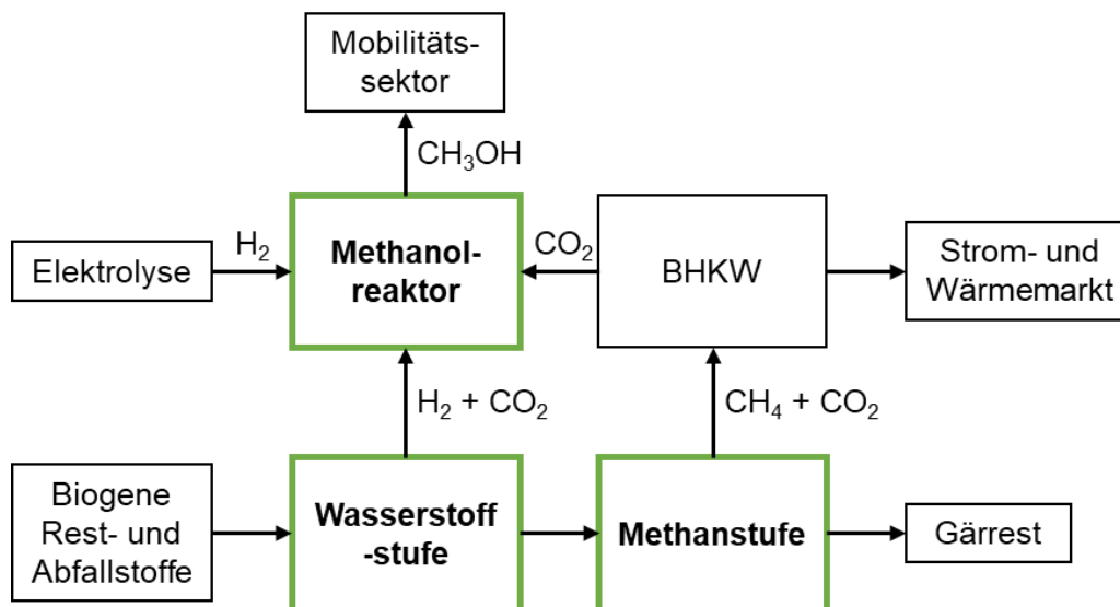
Abbildung 1: Schematisches Funktionsprinzip „BioMeth“ (Quelle: DBI)
